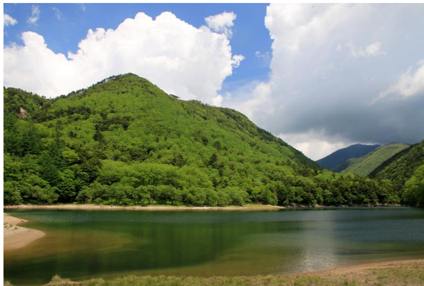
Lake Kirikomi and Lake Karikomi
